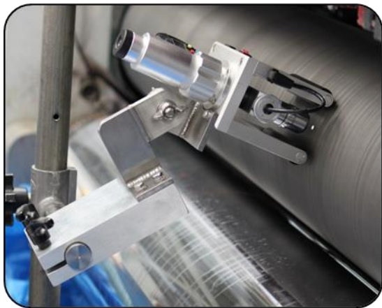
アニロックス・セル形状・深度・工学測定 セルチェックシステム・ミルで汚れの測定
